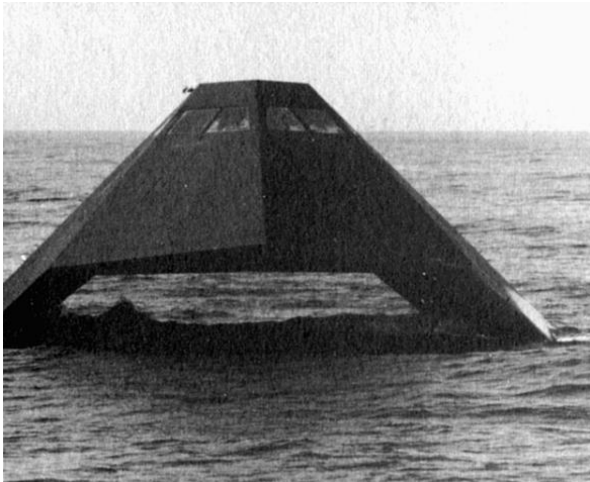
Малозаметный корабль во время испытаний недалеко от Западного побережья, середина 1980-х. (Фото Skunk Works )
