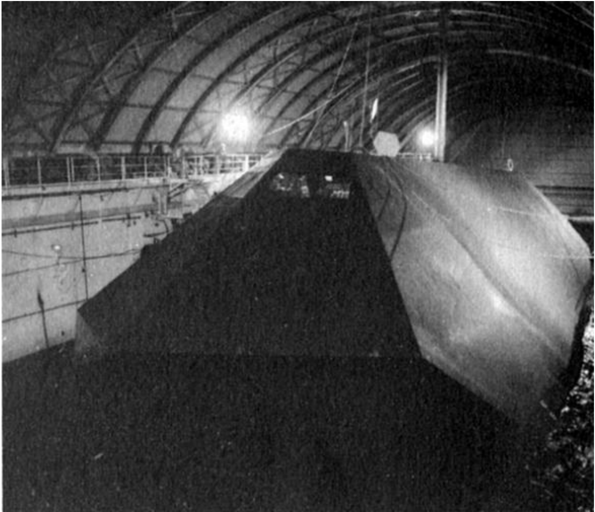
Малозаметный корабль внутри секретного плавучего дока, где производилась его окончательная сборка. (Фото Skunk Works )
